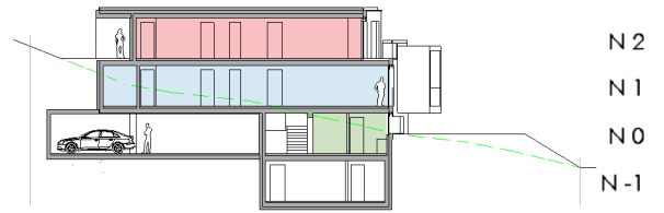
PRINZIPSCHNITT 1 : 500
